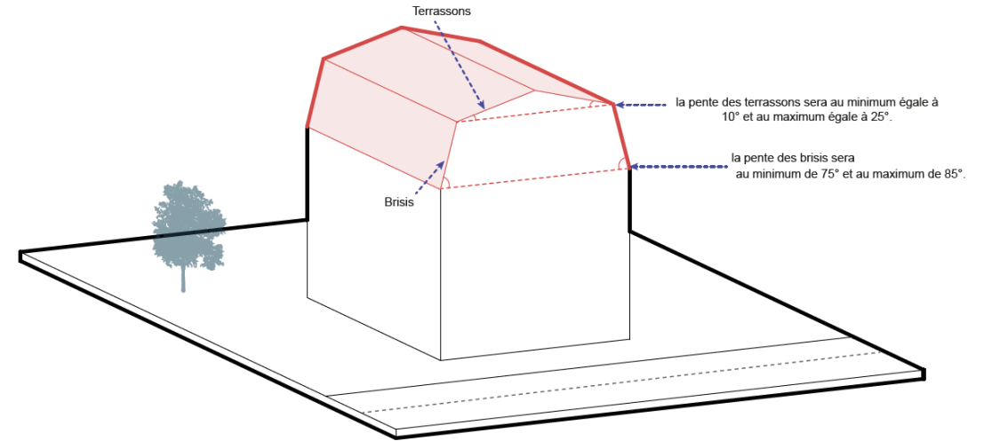
Toiture Mansart
