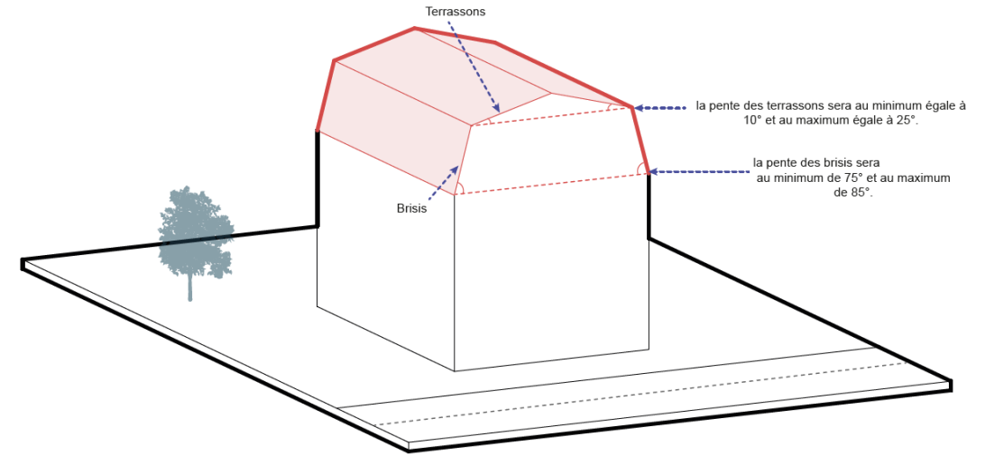
Toiture Mansart (R+1 seulement)
